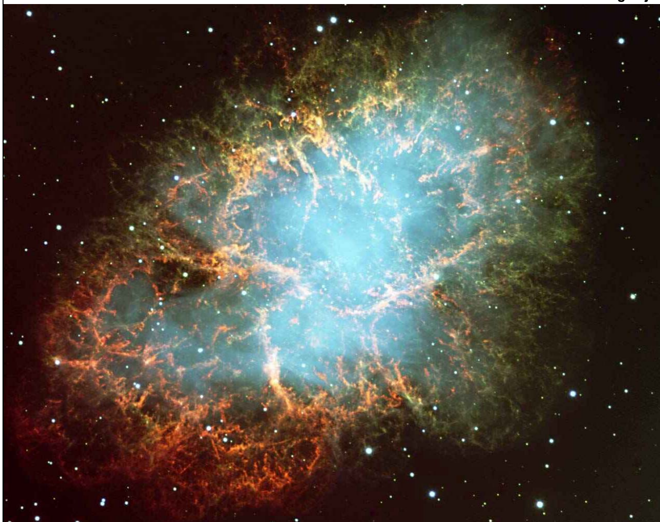
Nebulosa do Caranguejo
